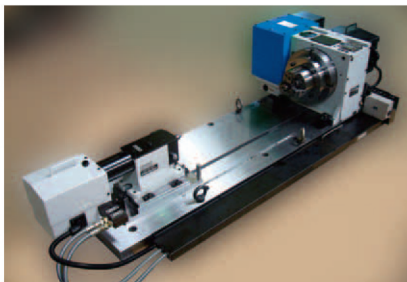
▲与尾部中心顶一同使用可以加工长尺寸工件
