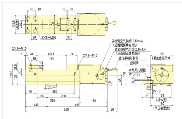
尺寸图
